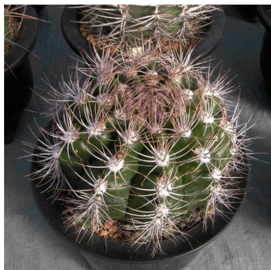
G. mostii v. immemoratum (活火山)
